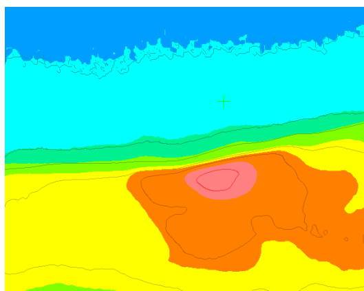
Rys. 17. Wykresy izoluksów dla żarówki N
