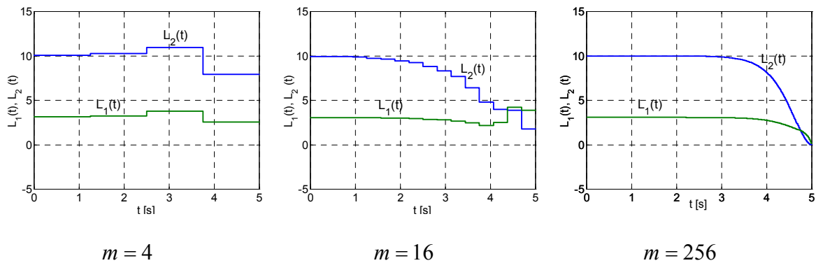
Rys.5. Optymalne współczynniki sprzężenia zwrotnego obliczone metodą rozkładu na falki Haara dla układu regulacji położenia kątownego anteny.
