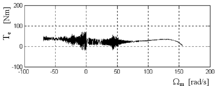
Fig.2. Motor reversal.
