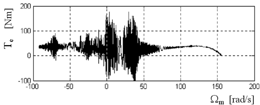
Fig.1. Motor reversal.
